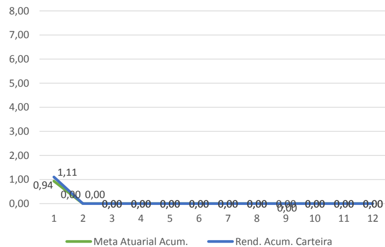
Meta Atuarial
